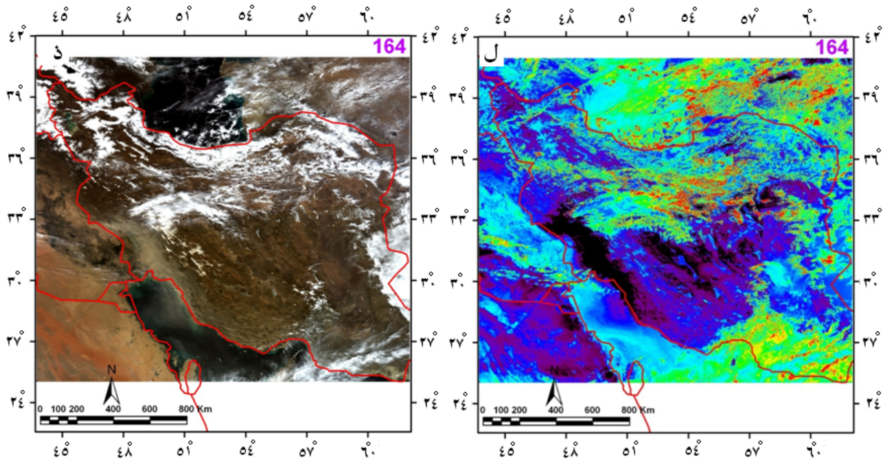
شکل ۸. تصویر گرد و غبار رنگی حقیقی ۱۳ ژوئن ۲۰۱۱ (ب) و بازسازی شده ۱۳ ژوئن ۲۰۱۱ (ا)
