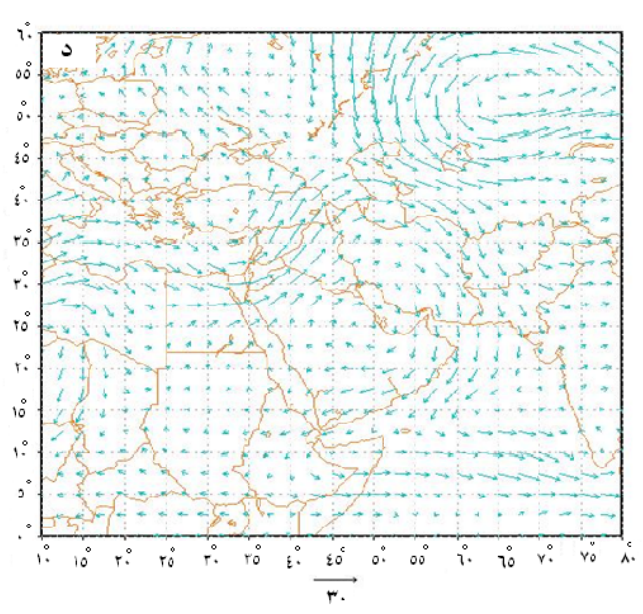
شکل ۱۰. جهت جریان باد در تراز ۱۰۰۰ میلی‌باری در ۱ ژوئن ۲۰۱۱ (ج) و جهت جریان باد در تراز ۵۰۰ میلی‌باری در ۱ ژوئن ۲۰۱۱ (د)
