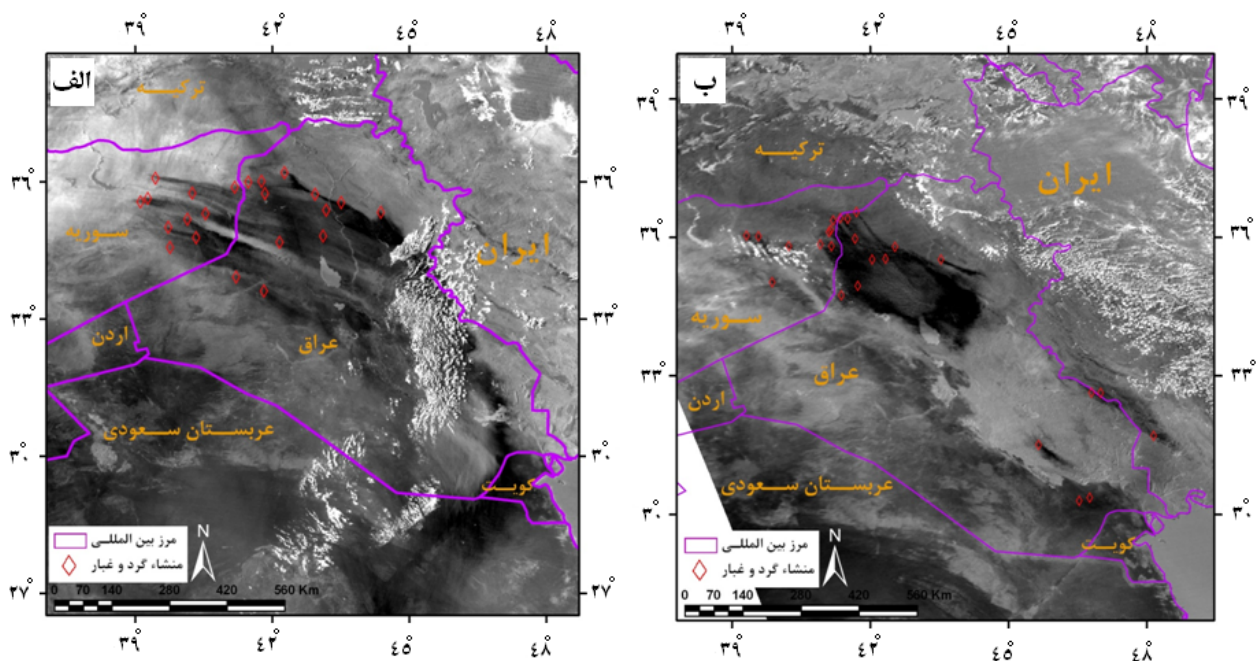
شکل ۳. تصویر منشاء گرد و غبار طوفان ۱ ژوئن ۲۰۱۱ (الف) و منشاء گرد و غبار طوفان ۱۱ ژوئن ۲۰۱۱ (ب)
