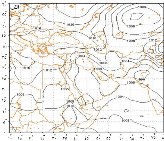
شکل ۹. فشار تراز دریا ۱ ژوئن ۲۰۱۱ (الف) و ارتفاع ژئوپتانسیل تراز ۵۰۰ میلی‌باری ۱ ژوئن ۲۰۱۱ (ب)
