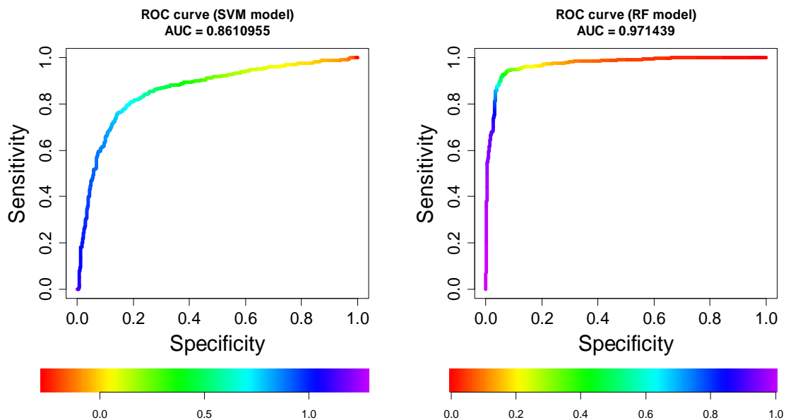
شکل ۱۱. ارزیابی دقت مدل‌های مورد بررسی با استفاده از سطح زیر نمودار (AUC)
