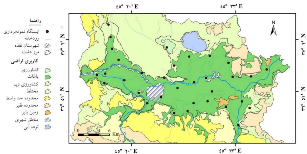
شکل ۷. نقشه کاربری اراضی محدوده مطالعاتی نقده
