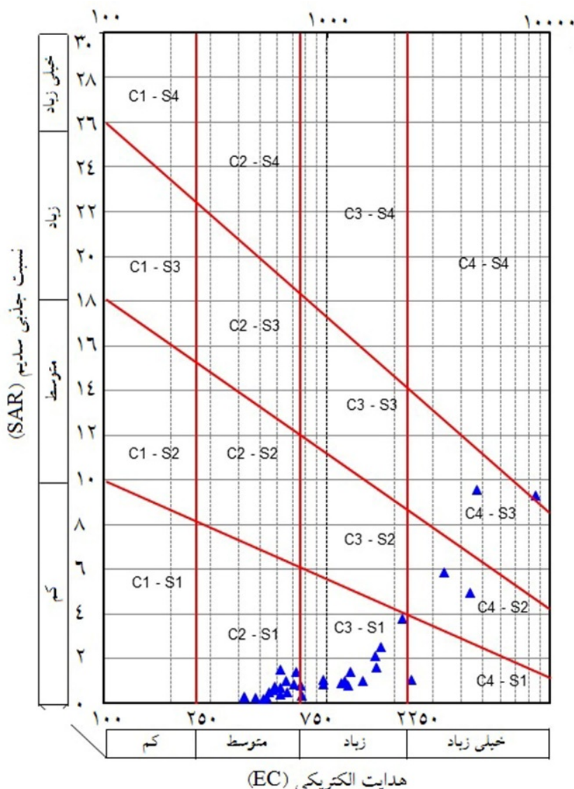
شکل ۵. توزیع نمونه‌ها در نمودار طبقه‌بندی کیفی کشاورزی ویلکاکس هدایت الکتریکی (EC)
