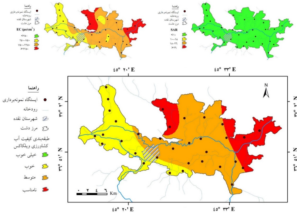
شکل ۶. نقشه پهنه‌بندی کیفی منابع آب زیرزمینی دشت نقده جهت مصارف کشاورزی
