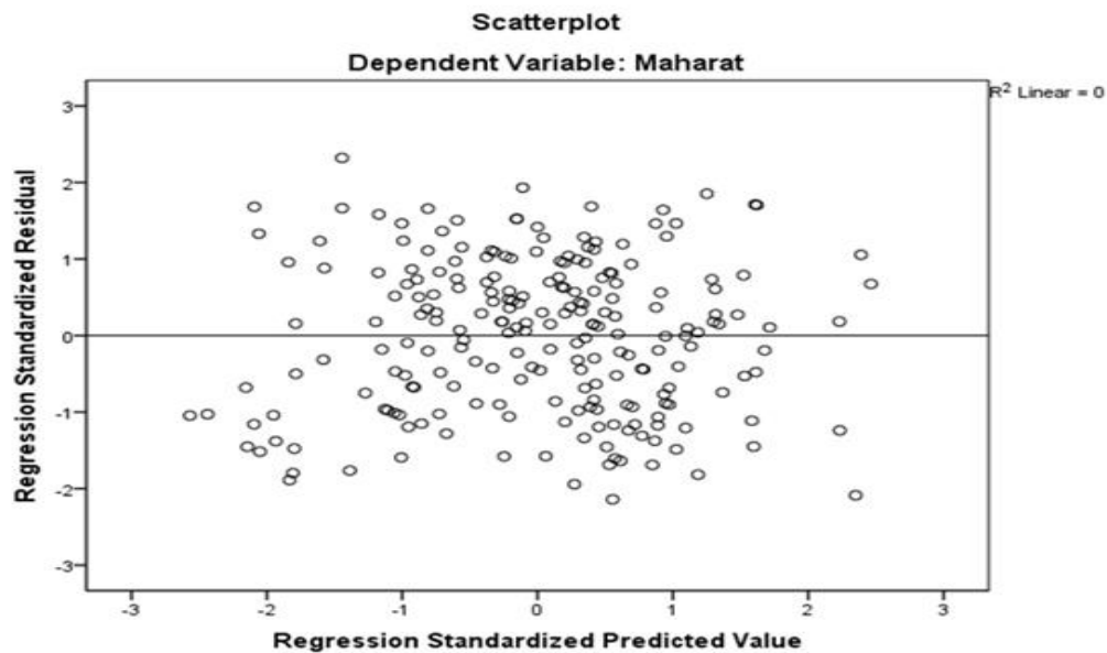
نمودار ۱. نمودار پراکندگی واریانس استاندارد شده خطاها
