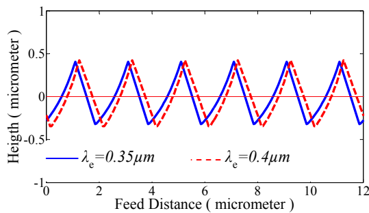
شکل (۹): اثر حداقل ضخامت براده و جنس قطعه کار بر زبری سطح ایجاد شده ( r_e = 3 \mu m )
