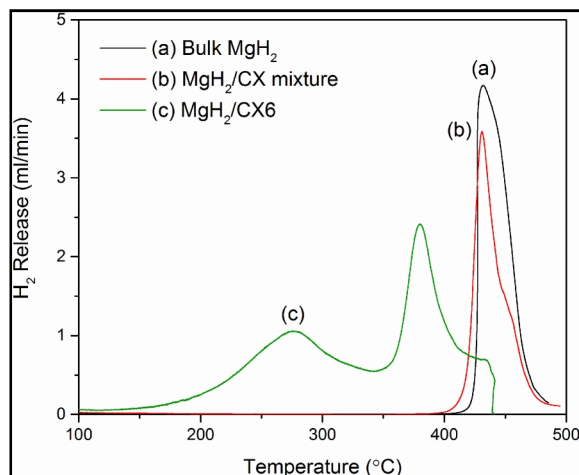
شکل ۵: منحنی رهایش هیدروژن (TPD) برای (a) پودر منیزیم Bulk MgH 2 ، (b) مخلوط فیزیکی ۱۰ wt.% MgH 2 /CX و (c) نانوکامپوزیت ۱۰ wt.% MgH 2 /CX6 mixture.
