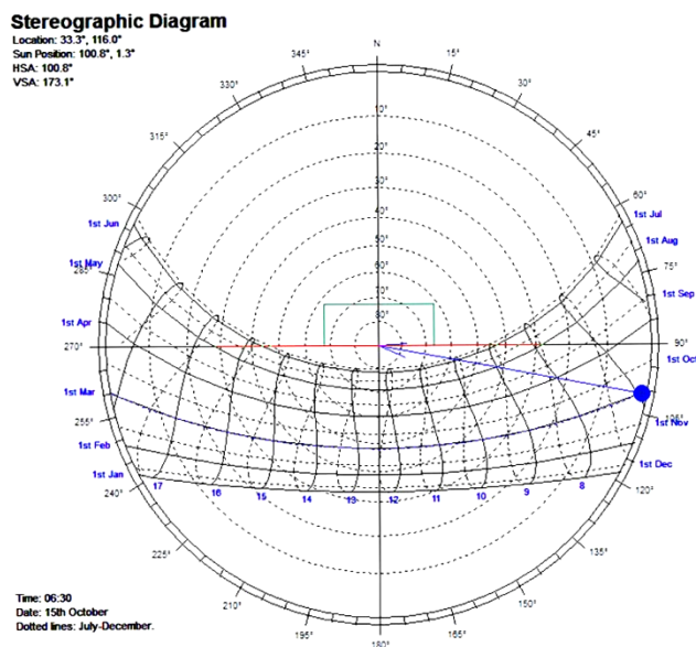
شکل ۳. نمودار خورشیدی
