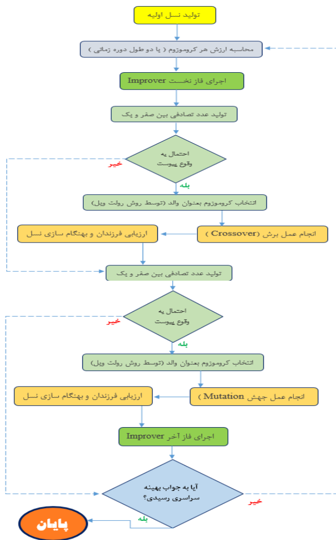
شکل ۶- ساختار الگوریتم ژنتیک بهبود دهنده تطبیق پذیر (ژبت)
