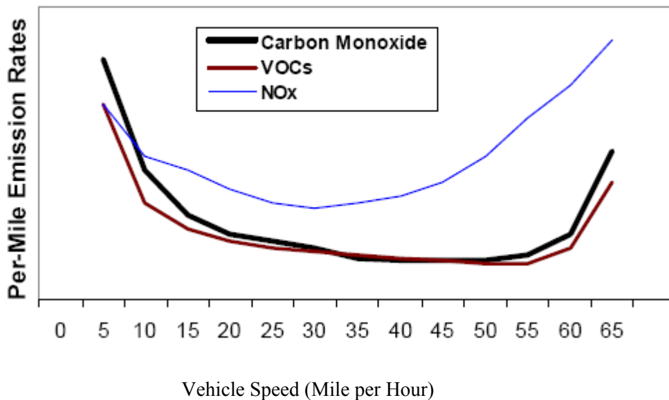
نمودار ۱- ارتباط بین میزان انتشار آلاینده‌ها با سرعت وسیله نقلیه (۷)
