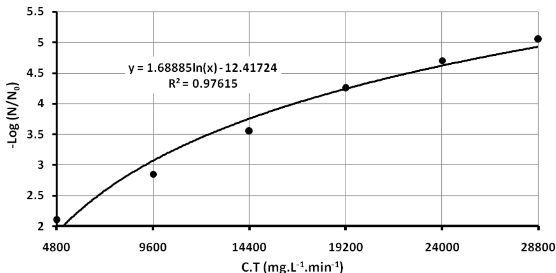
شکل ۲- رابطه میان C.T Value و کلیفرم های مدفوعی غیر فعال شده پساب HRF در تماس با محلول H_2O_2-Ag^+
