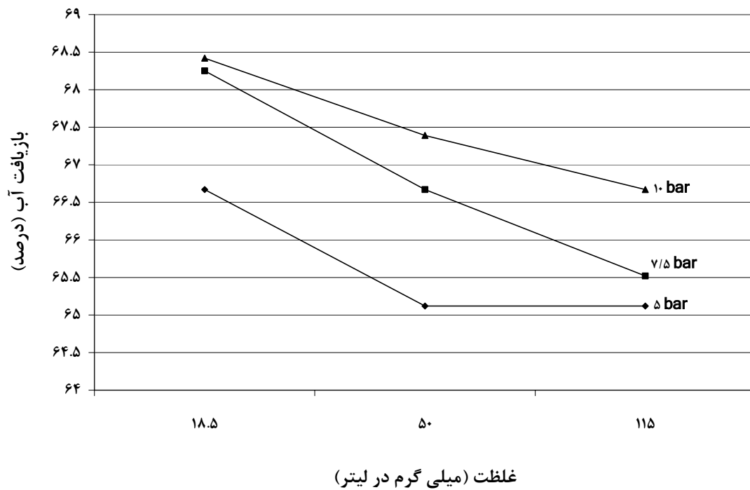
نمودار ۴- اثر غلظت نیکل در فاضلاب ورودی بر روی بازیافت آب
