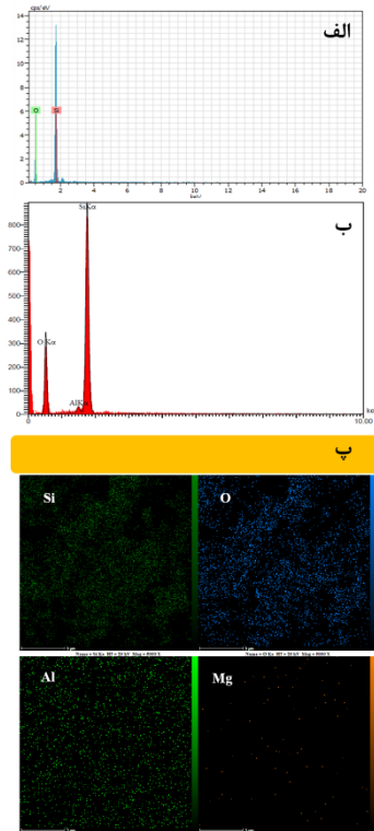
شکل ۳- نتایج آنالیز EDS (الف) سیلیس و (ب) زئولیت ZSM-12 و نتایج MAP (پ) نانوجندسازه Figure 3. EDX result of (a) silica, (b) ZSM-12 zeolite, and MAP result of (c) nanocomposite
