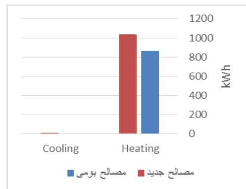
شکل ۱۵- مقایسه مصرف انرژی با مصالح بومی و جدید Figure15- Comparison between the amount of energy consumption using traditional and new materials
