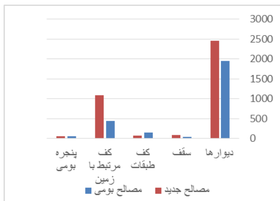
شکل ۱۶- مقایسه تبادل حرارتی سالانه سطوح مختلف Figure16- Comparison between the amount of thermal exchange
