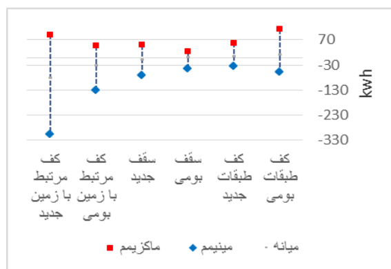
شکل ۱۷- بازه تبادل حرارتی سالانه سطوح افقی Figure17- The range of annual energy exchange from horizontal surfaces
