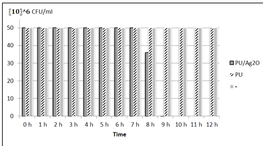
نمودار ۱- تاثیر نانوکامپوزیت PU/Ag 2 O بر رشد باکتری اشیریشیاکلی با گذشت زمان
