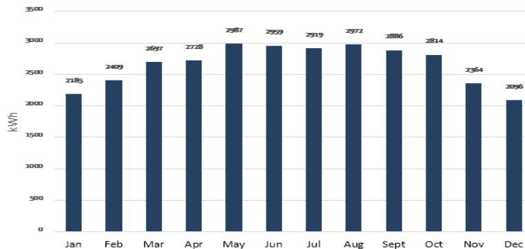
شکل ۱۰ - انرژی خالص خروجی ماهانه Figure 10 – Monthly output pure energy
