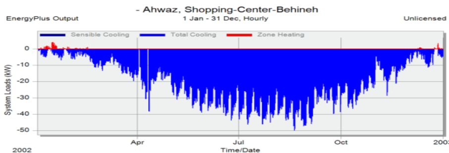
شکل ۸- نتایج ساعتی تفکیکی بارهای سرمایشی و گرمایشی ساختمان
