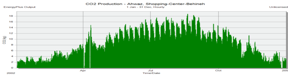
شکل ۹ - نتایج ساعتی تولید CO 2 Figure 9- Hourly results of CO 2 production
