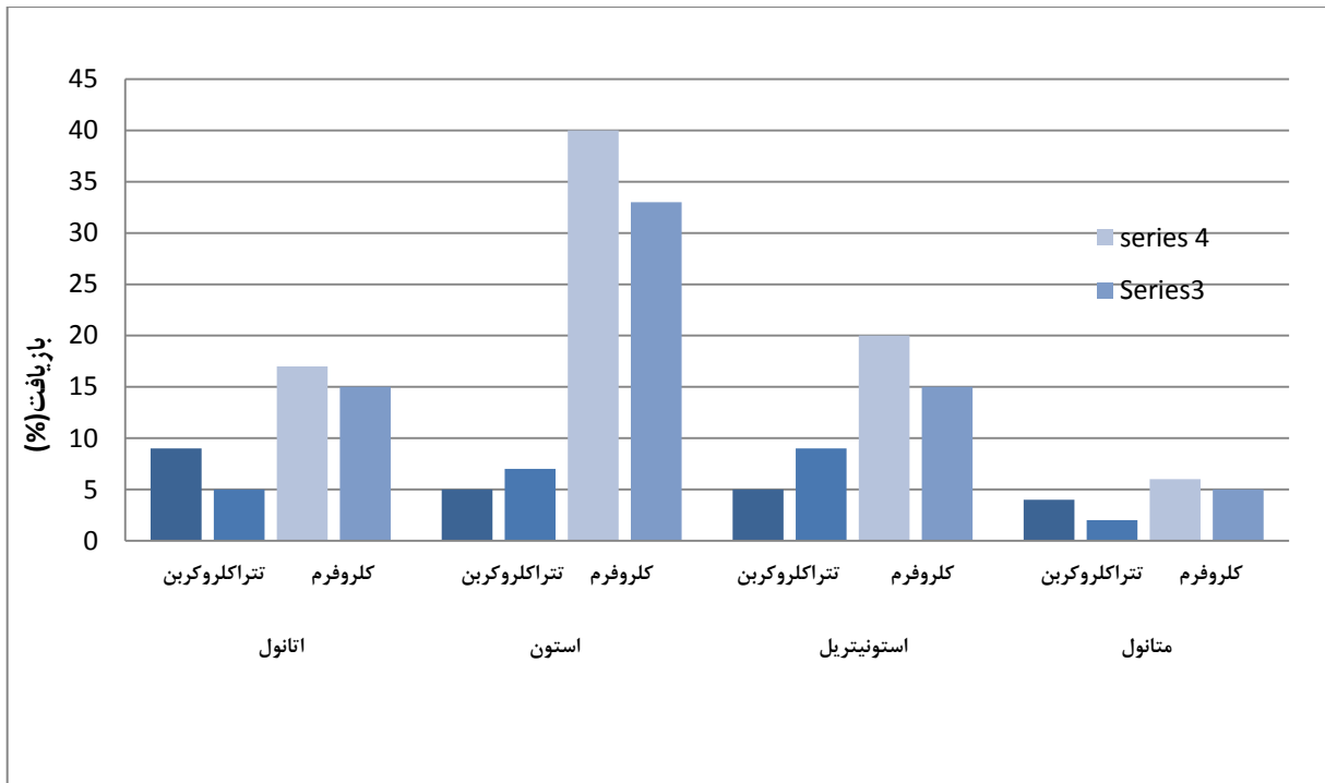
شکل ۱- انتخاب بهترین محلول استخراج کننده و پخش شونده برای روش میکرواستخراج مایع - مایع پخشی در شرایط: حجم نمونه، ۵mL؛ حجم محلول پخش شونده، ۱mL؛ حجم محلول استخراج کننده، ۱۰۰mL (بدون در نظر گرفتن شرایط اپتیمم بلکه فقط برای انتخاب جفت محلول مناسب برای مراحل بعد).
