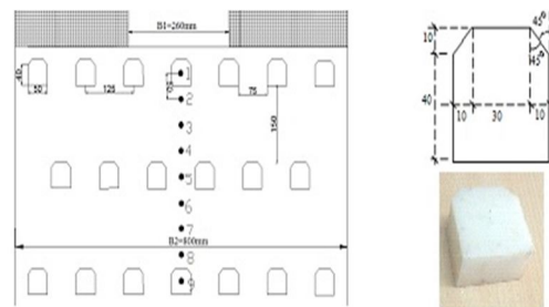
شکل ۲. شکل و ابعاد زبری‌ها و نحوه آرایش در بستر حوضچه (ابعاد به میلی‌متر می‌باشد)
