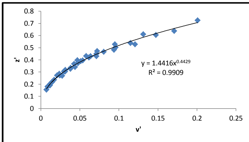
شکل ۴- حصول مقادیر A_2 و n_2
