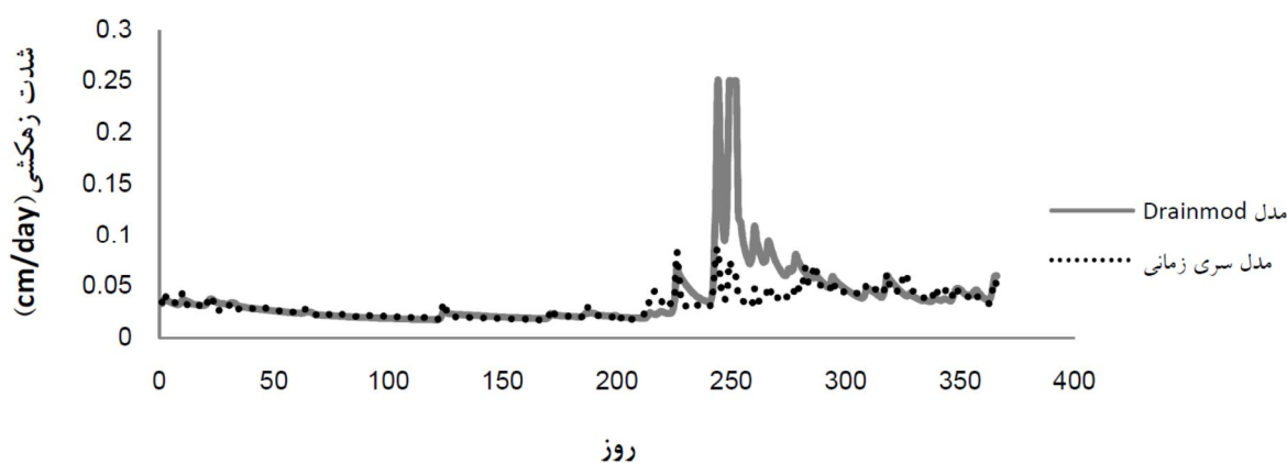
شکل ۱. توسعه مدل ARMAX(1,2,0) روی داده‌های شدت تخلیه زهاب
