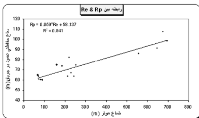
شکل ۱۷: نمودار همبستگی بین شعاع موثر و شعاع حفاظتی عمود بر جریان
