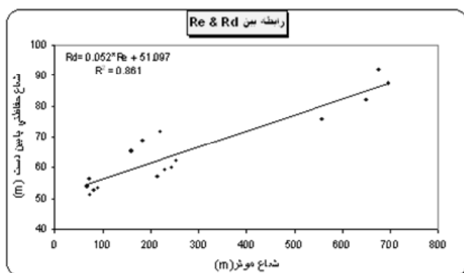
شکل ۱۶: نمودار همبستگی بین شعاع موثر و شعاع حفاظتی پایین دست
