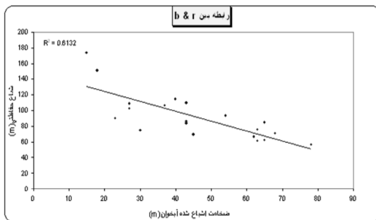
شکل ۱۳: نمودار همبستگی بین ضخامت اشعاع شده آبخوان و شعاع حفاظتی بالادست جریان
