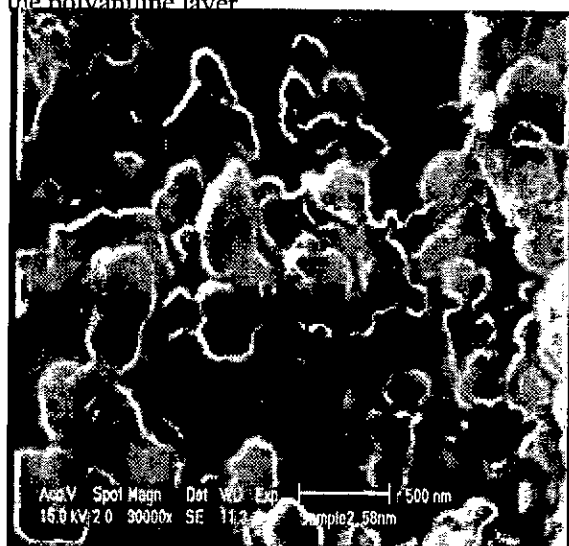
Fig. 2. SEM images of the Pt-Ru/PAN nanocomposite.
