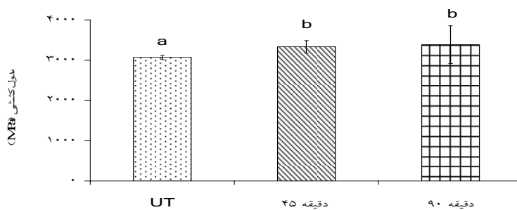
شکل ۳. اثر مستقل زمان تیمار قلبی آرد کاه برنج بر مدول کششی چندسازه
