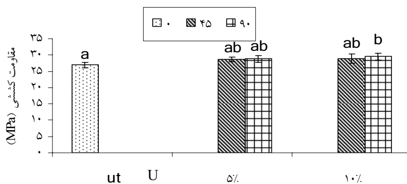
شکل ۸. تاثیر متقابل غلظت و زمان تیمار قلیایی آرد کاه برنج بر مقاومت کششی چندسازه
