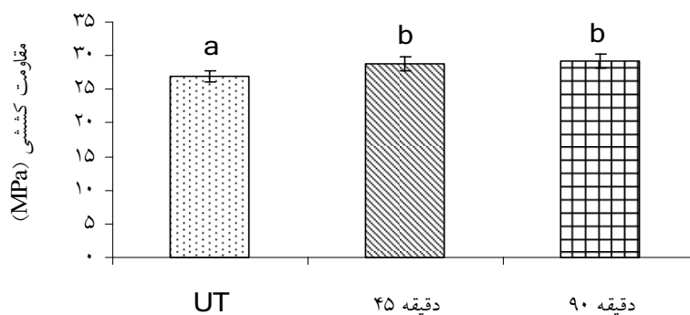
شکل ۷. اثر مستقل زمان تیمار قلیایی آرد کاه برنج بر مقاومت کششی چندسازه
