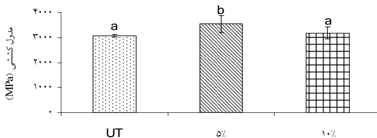
شکل ۱. تاثیر تیمار قلبی آرد کاه برنج بر مدول کششی چندسازه
