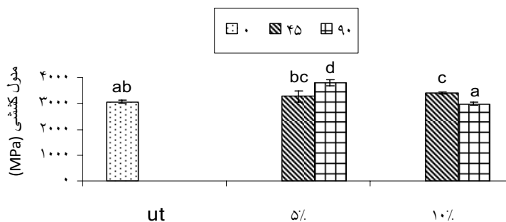
شکل ۴. اثر متقابل غلظت و زمان تیمار قلبی آرد کاه برنج بر مدول کششی چندسازه
