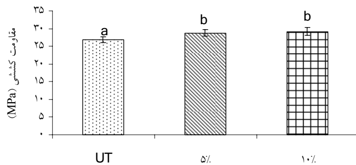
شکل ۶. اثر مستقل غلظت تیمار قلیایی آرد کاه برنج بر مقاومت کششی چندسازه
