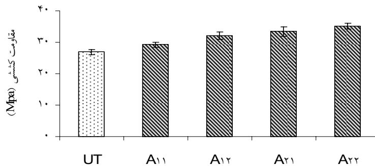
شکل ۵. تاثیر تیمار قلیایی آرد کاه برنج بر مدول کششی چندسازه
