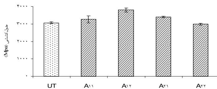
شکل ۲. اثر مستقل غلظت تیمار قلبی آرد کاه برنج بر مدول کششی چندسازه
