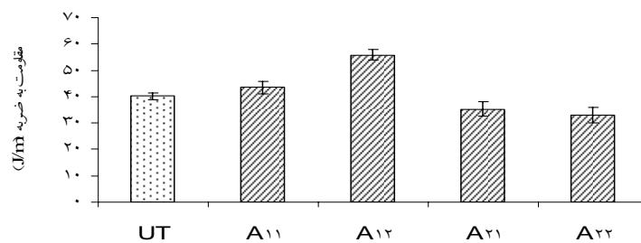
شکل ۹. تاثیر تیمار قلیایی آرد کاه برنج بر مقاومت به ضربه چندسازه
