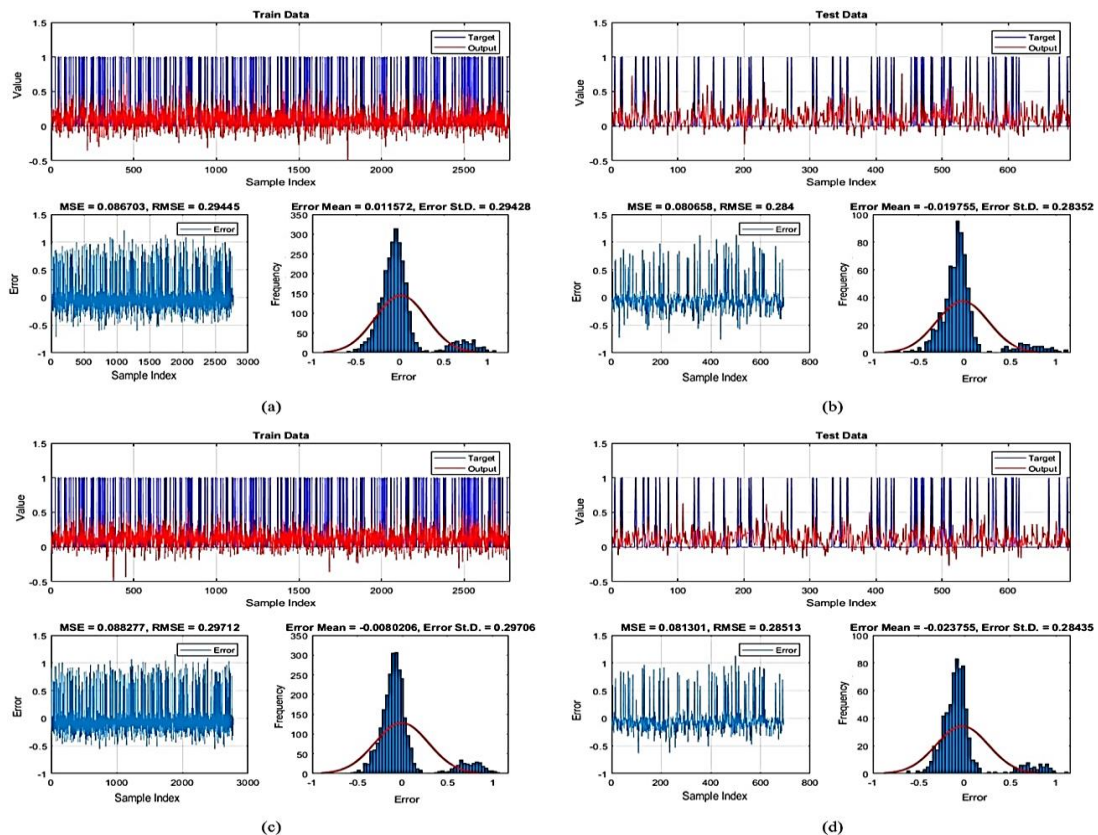
شکل ۷: مقادیر MSE, RMSE, Error Mean, Error STD
