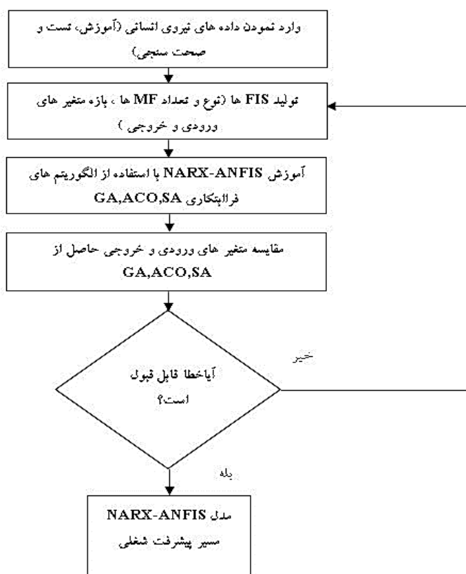
شکل ۴: فلوچارت مدل
