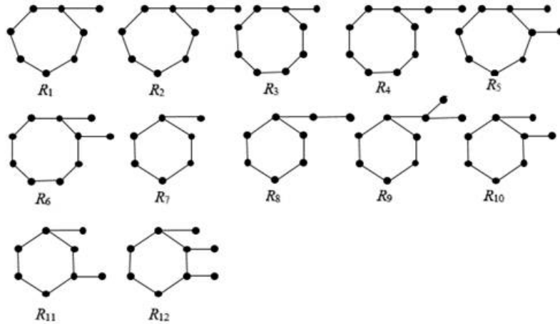
شکل ۳- خانواده \mathcal{R}
