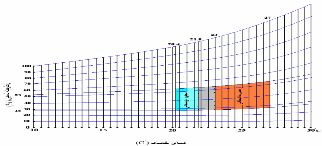
شکل ۴: جدول زیست-اقلیمی آسایش حرارتی در تابستان و زمستان برای شهر یزد مأخذ: نگارندگان
