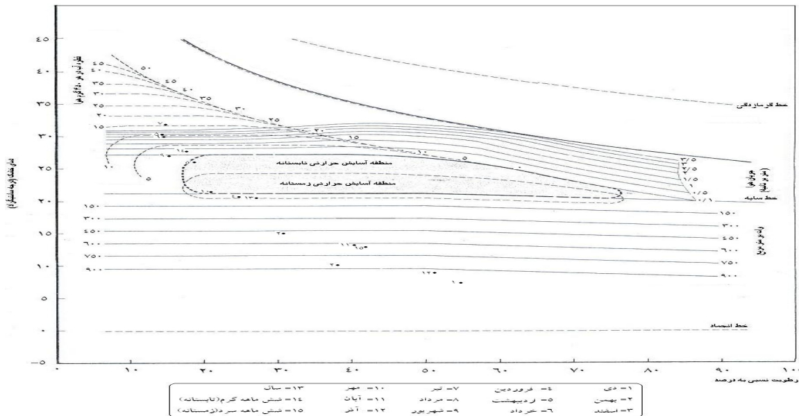
شکل ۳: نمودار زیست-اقلیمی اولگی (Olgay, 1973) وضعیت آسایش حرارتی ایستگاه یزد به تفکیک ماهانه مأخذ: نگارندگان
