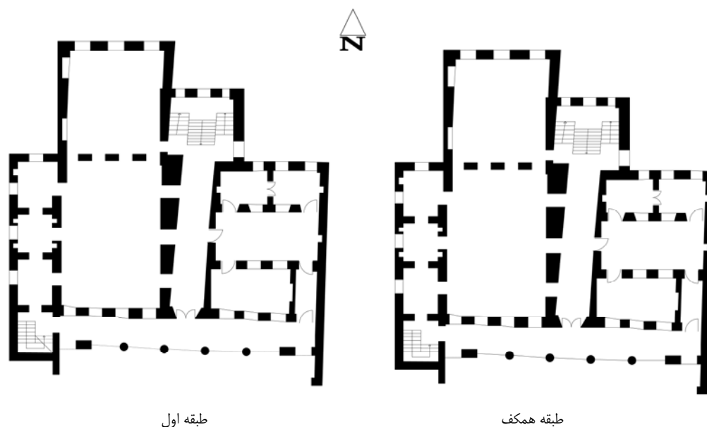
شکل ۴. پلان طبقات خانه امیربهادر
