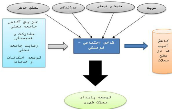
شکل ۱. چهارچوب نظری و مدل مفهومی توسعه پایدار محله‌ای
