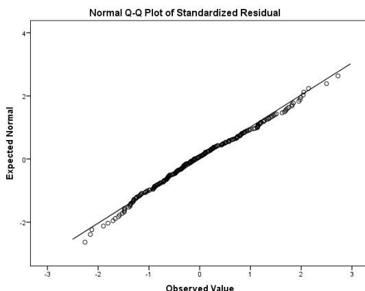
نمودار ۱. منحنی احتمال نرمال در مدل پیش بینی گرایش به اعتیاد
