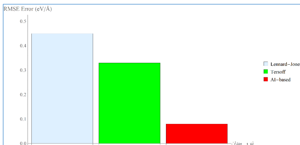
شکل ۱: مقایسه خطای جذر ریشه میانگین مربعات برای میدان‌های نیروی مختلف در پیش‌بینی انرژی
