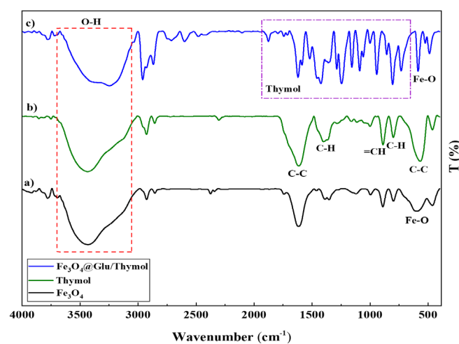
شکل ۲. طیف FT-IR تیمول، \text{Fe}_3\text{O}_4 و نانوذرات \text{Fe}_3\text{O}_4@\text{Glu-Thymol} . وجود پیک‌های مربوط به هر دو ماده سازنده در ساختار نانوذرات \text{Fe}_3\text{O}_4@\text{Glu-Thymol} نشان دهنده سنتز صحیح آنان است.
