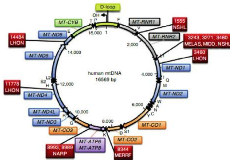
شکل ۳: نقشه فیزیکی mtDNA در انسان (Amorim et al., 2019)
