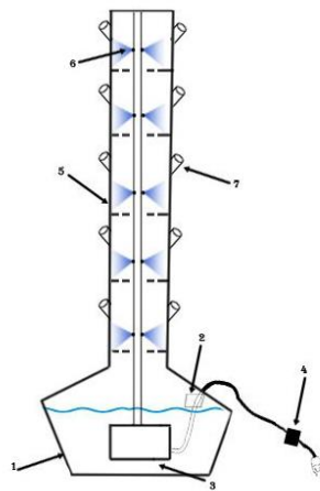
شکل ۱- طرحواره سامانه اروپونیک عمودی شامل: ۱- مخزن ۲- درب مخزن ۳- پمپ ۴- تایمر ۵- ستون سامانه و طبقات ۶- نازل های ۳۶۰ درجه ۷- محل قرارگیری گلدان های نگهدارنده گیاه توت فرنگی
