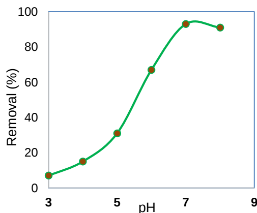
شکل ۷: تأثیر pH محلول بر میزان جذب یون‌های \text{Zn}^{2+} توسط نانوجاذب.
