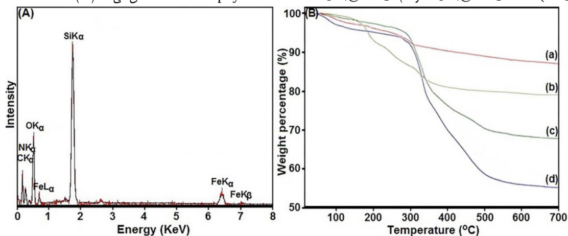
شکل ۳۵: آنالیز EDX نانوذرات (B, \text{Fe}_3\text{O}_4/\text{SiO}_2\text{-TCT-Theophylline} ) آنالیز TGA نانوذرات (a, \text{Fe}_3\text{O}_4/\text{SiO}_2\text{-NH}_2 (b), \text{Fe}_3\text{O}_4/\text{SiO}_2\text{-TCT-(CH}_2)_3\text{Br} (c) و \text{Fe}_3\text{O}_4/\text{SiO}_2\text{-TCT-Theophylline} (d) (۲۸).
