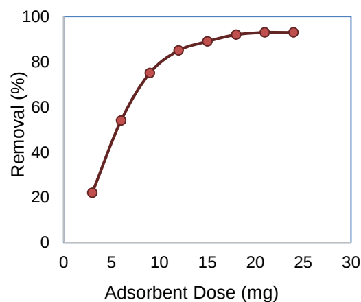
شکل ۶: بهینه‌سازی دوز نانوجاذب در حذف یون‌های \text{Zn}^{2+} .
