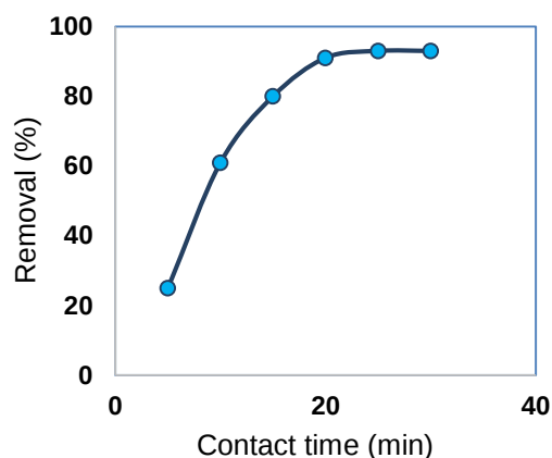
شکل ۹: بهینه‌سازی زمان تماس نانوجاذب \text{Fe}_3\text{O}_4@\text{SiO}_2 -TCT-Theophylline در جذب یون‌های \text{Zn}^{2+} .
