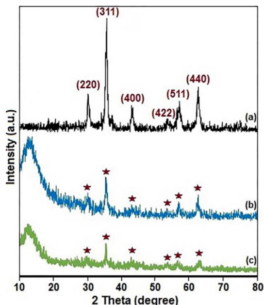
شکل ۲: پراش اشعه X نانوذرات سنتزی (a) \text{Fe}_3\text{O}_4 ، (b) \text{Fe}_3\text{O}_4@ \text{SiO}_2 و (c) \text{Fe}_3\text{O}_4@ \text{SiO}_2 -TCT-Theophylline (۲۸).
