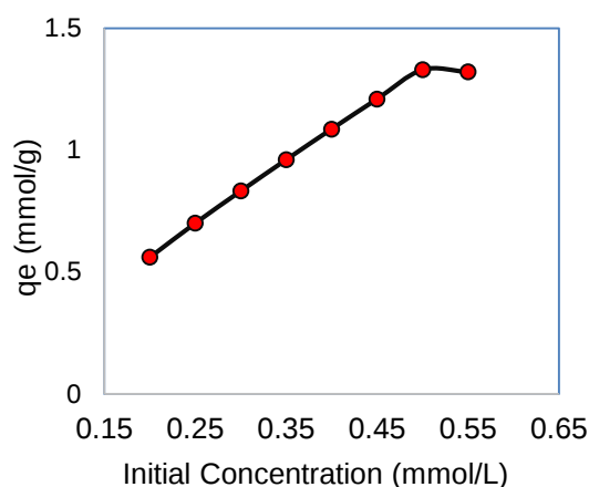
شکل ۸: بهینه‌سازی غلظت اولیه یون‌های \text{Zn}^{2+} در حضور نانوجاذب \text{Fe}_3\text{O}_4@\text{SiO}_2 -TCT-Theophyllin.
