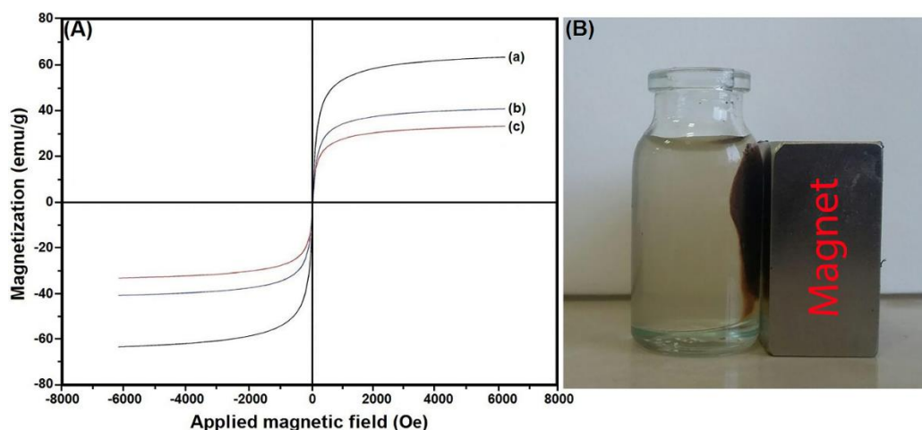
شکل ۵: نمودارهای VSM نانوذرات (a) \text{Fe}_3\text{O}_4 (b) \text{Fe}_3\text{O}_4@ \text{SiO}_2 و (c) \text{Fe}_3\text{O}_4@ \text{SiO}_2\text{-TCT-Theophylline} (B) جداسازی نانوجاذب با استفاده از مگنت مغناطیسی (۲۸).
