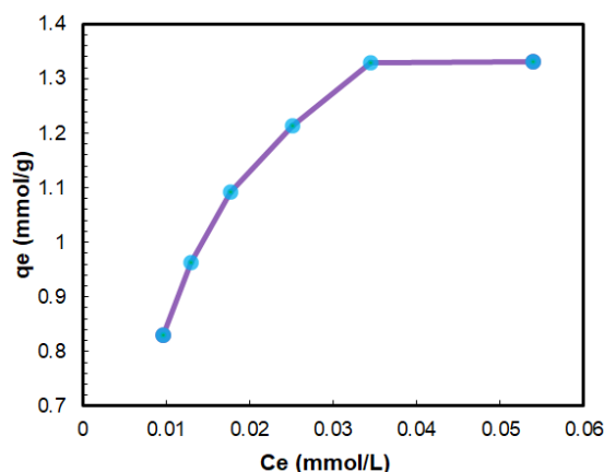
شکل ۱۰: ایزوترم‌های جذب یون‌های \text{Zn}(\text{II}) توسط نانوجاذب \text{Fe}_3\text{O}_4@\text{SiO}_2 -TCT-Theophylline.
