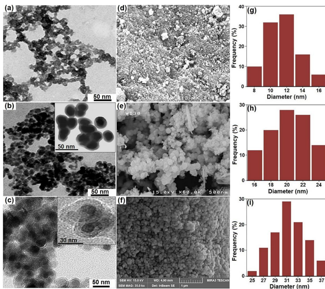
شکل ۳: تصاویر TEM نانوذرات (a) Fe_3O_4 (b) Fe_3O_4@SiO_2 (c) Fe_3O_4@SiO_2-TCT-Theophylline و تصاویر FE-SEM نانوذرات (d) Fe_3O_4 (e) Fe_3O_4@SiO_2 (f) Fe_3O_4@SiO_2-TCT-Theophylline و تصاویر DLS نانوذرات (g) Fe_3O_4 (h) Fe_3O_4@SiO_2 (i) Fe_3O_4@SiO_2-TCT-Theophylline .
