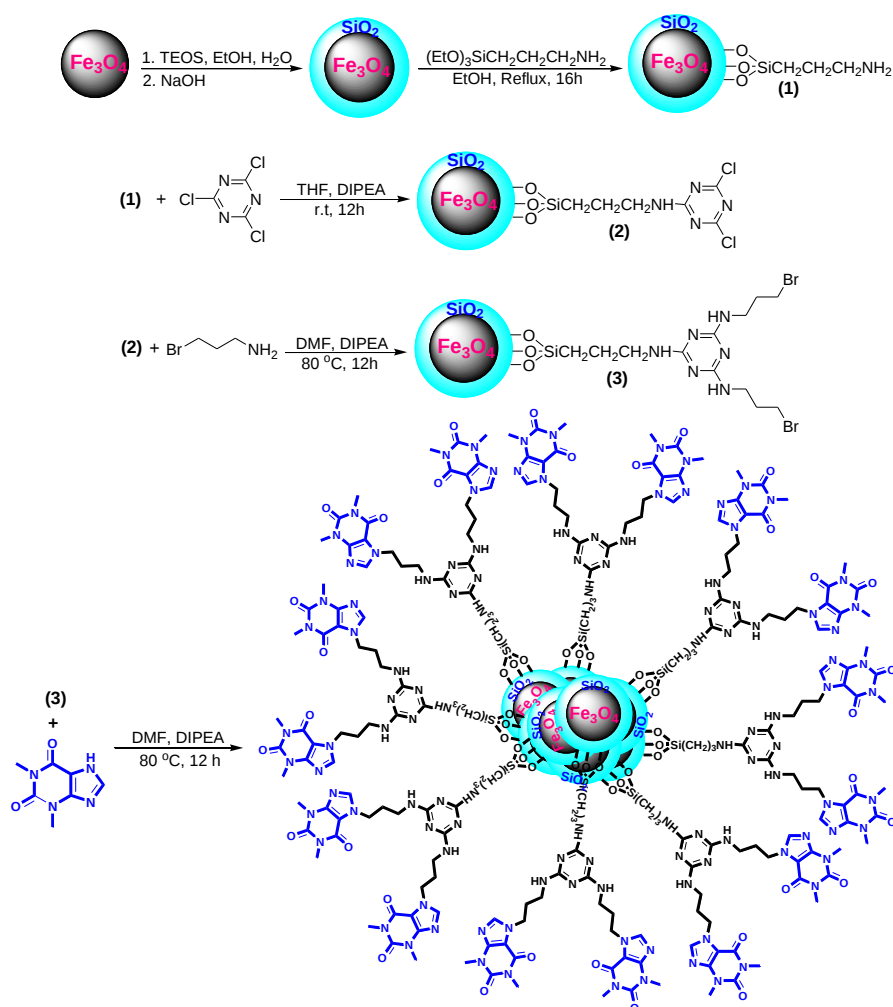
طرح ۱: فرآیند سنتز و عامل دار شدن نانوذرات هسته-پوسته \text{Fe}_3\text{O}_4@\text{SiO}_2 با مولکول های تئوفیلین (۲۸).
