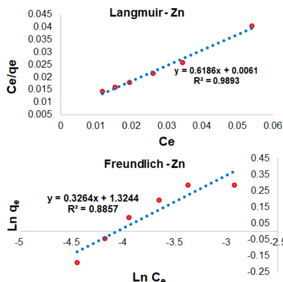
شکل ۱۱: منحنی‌های ایزوترم با مدل‌های لانگمویر و فرنللیچ در جذب یون‌های Zn(II).
