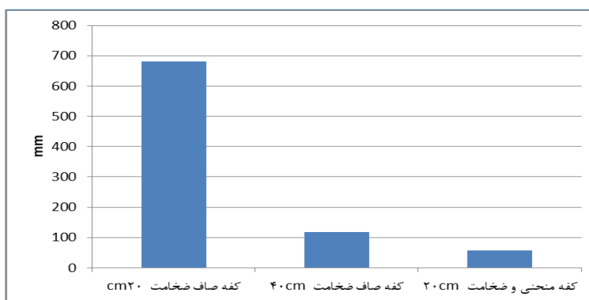
شکل ۸: مقادیر تغییر شکل بیشینه در موارد مطالعه بر روی سطح زمین
