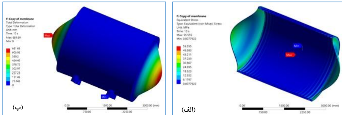
شکل ۳: میزان تنش و تغییر شکل در مخزن با کفه‌های تخت با ضخامت ۲۰ سانتی‌متر بر روی زمین
