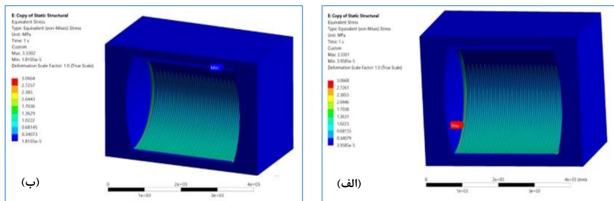
شکل ۷: میزان توزیع تنش در مخزن با کفه منحنی مدفون (الف) مدول یانگ ۷۹۳ مگاپاسکال (ب) مدول یانگ ۲۰۰ مگاپاسکال
