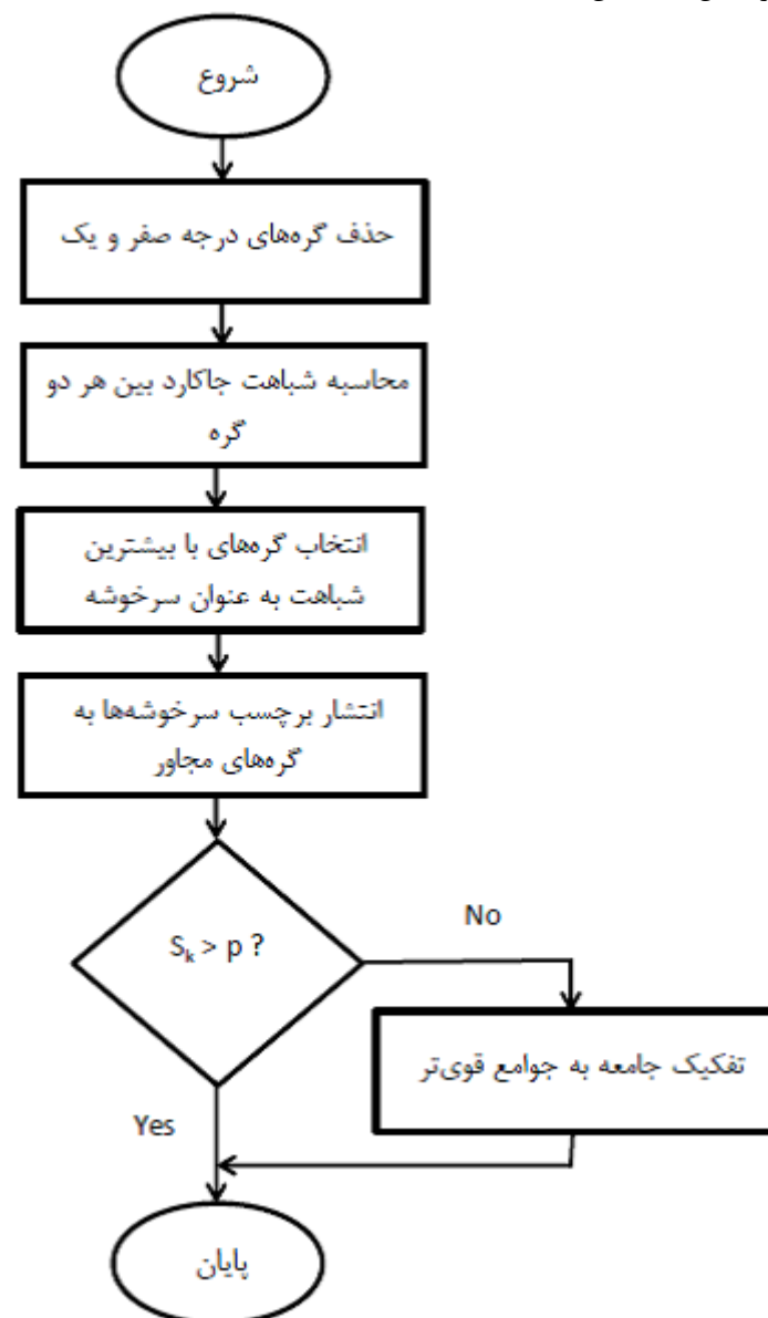
شکل ۳. فلوچارت روش پیشنهادی Figure 3. Flowchart of the proposed method
