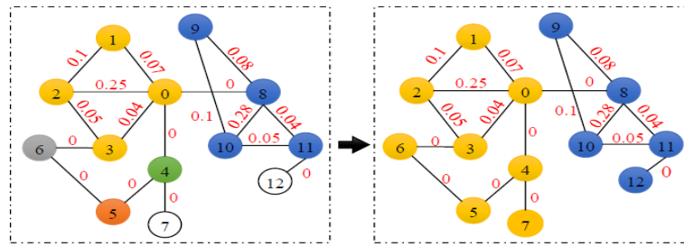
شکل ۲. نمونه‌ای از فرایند شناسایی جوامع براساس الگوریتم LBLD [۱]
