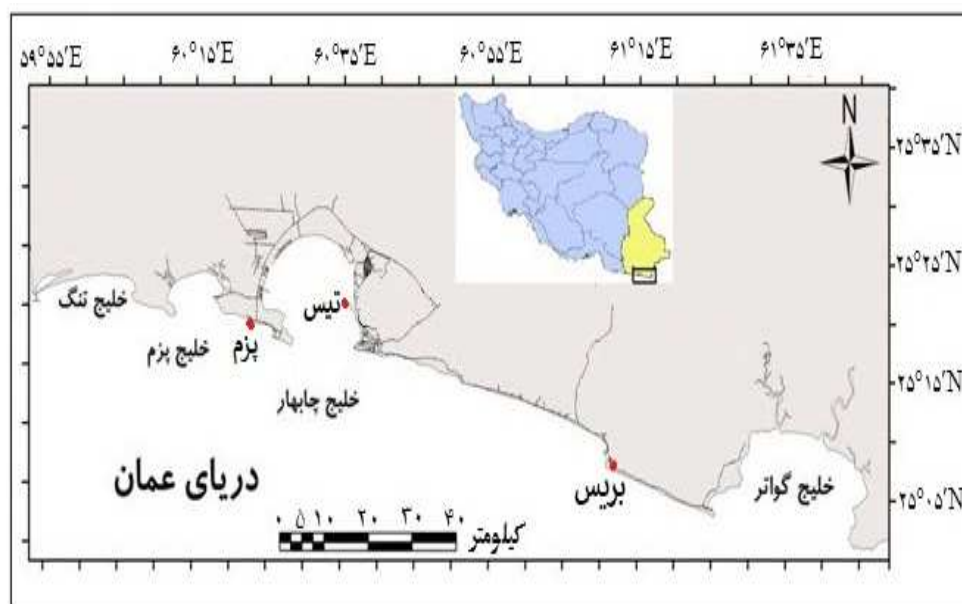
شکل ۱- موقعیت جغرافیایی ایستگاه‌های نمونه‌برداری خرچنگ شناگر آبی
