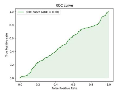
MVSA-Single-PCA
