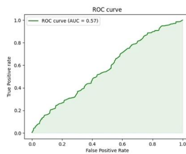
MVSA-Single-SVD
