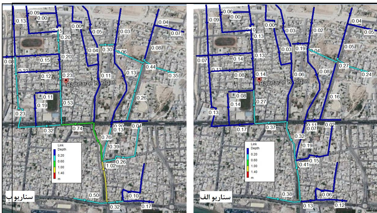
تصویر ۲- تغییرات عمق جریان در سطح شبکه اصلی در دو شرایط کرانی سناریو الف و ب - (ترسیم: نگارندگان، ۱۳۹۸).
