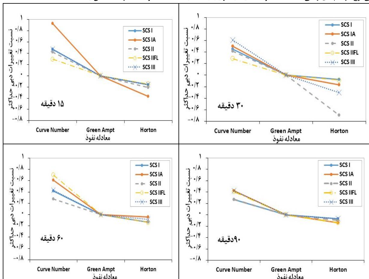
تصویر ۵- درصد تغییرات دبی حداکثر رواناب نسبت به معادلات نفوذ انتخابی، برای شرایط انتخاب روش روندیابی موج سینماتیک و گام‌های زمانی ۱۵، ۳۰، ۶۰ و ۹۰ دقیقه- (ترسیم: نگارندگان، ۱۳۹۸).
