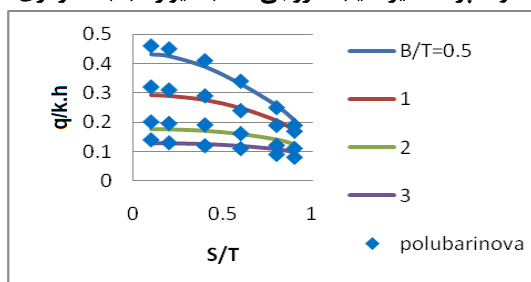
شکل ۱۴- مقایسه بدهی نشت از زیر سد ناتراوا با سپر ورقه ای قرینه واقع بر پی همگن با ژرفای متناسبی با نتایج پولوبارینووا- کوچینا.
