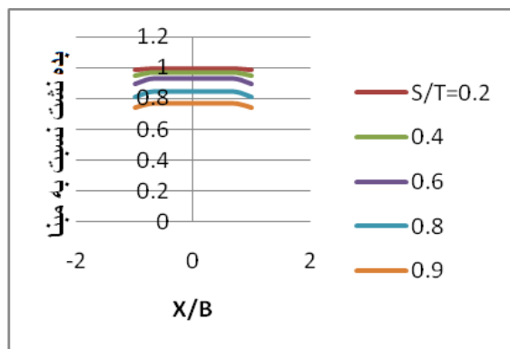
شکل ۵- اثر موقعیت دیواره‌ی آب بند بر بدهی نشت نسبت به مبنا از زیر سدهای ناتراوا واقع بر پی همگن ( B/T=3 ).
