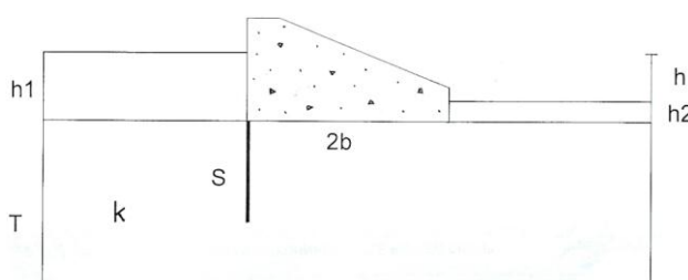
شکل ۱- شبیه ریاضی سد ناتراوا واقع بر پی همگن با پرده‌ی آب بند بالا دست.
