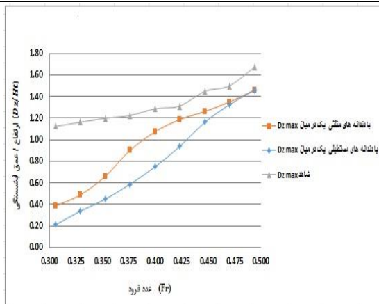
د- حداکثر عمق آبشستگی در سه حالت شاهد و با دندانهای مستطیلی و مثلثی یک در میان
