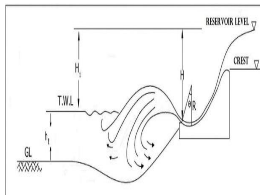
شکل ۱- طرح واره‌ی کلی آبشستگی در پائین
