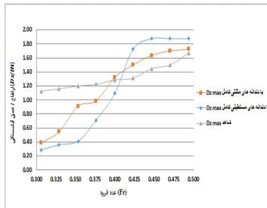
ج- حداکثر عمق آبشستگی در سه حالت شاهد و با دندانهای مستطیلی و مثلثی کامل
