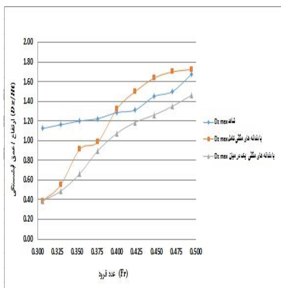
ب- حداکثر عمق آبشستگی در سه حالت شاهد و با دندان‌های مثلثی کامل و یک در میان
