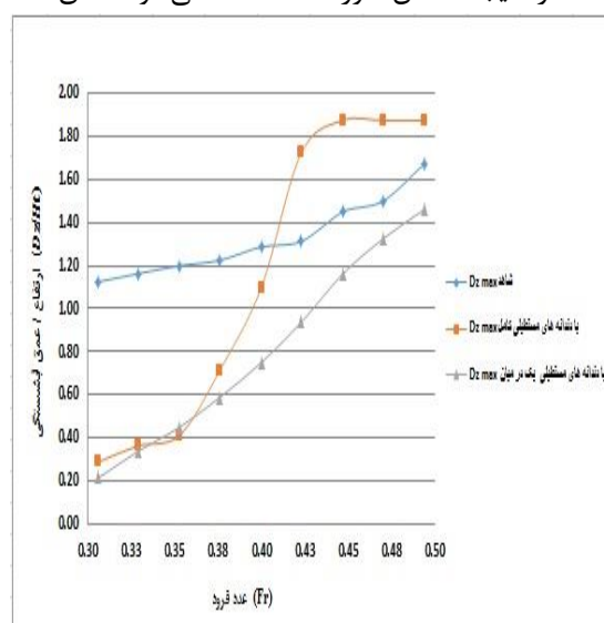
الف- حداکثر عمق آبشستگی در سه حالت شاهد و با دندان‌های مستطیلی کامل و یک در میان
