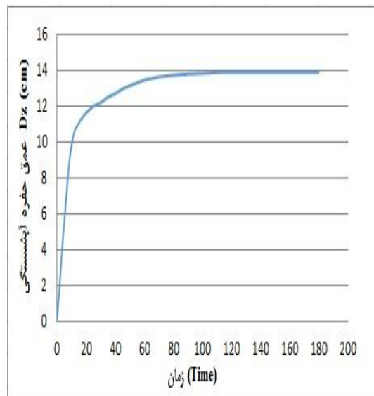
شکل ۶- نمودار زمان تعادل برای عمق آبستگي
