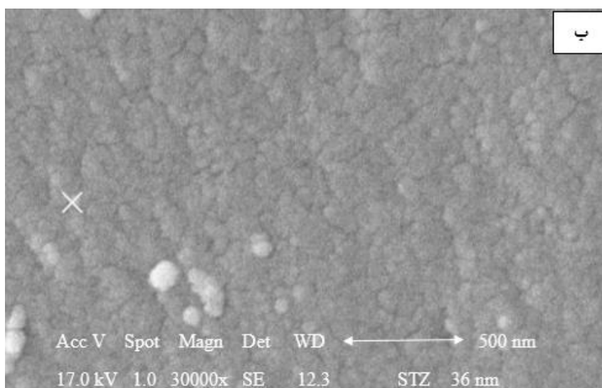
شکل ۴- تصاویر میکروسکوپ الکترونی روبشی و آنالیز انرژی تفکیکی (الف) اکسید روی خالص (Z) (ب) اکسید روی آلاینده شده با Si و Ti (STZ)
