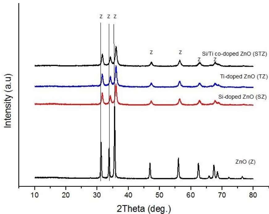
شکل ۱- الگوی تفرق اشعه ایکس نمونه خالص اکسید روی (Z) و آلانیده شده با Ti/Si کلسینه شده در دمای 450^{\circ}\text{C}
