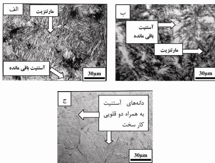
شکل ۴- تصویر SEM از ریزساختار میکروسکوپی لایه‌های گوناگون رسوبی پس از آزمون سایش الف- لایه‌ی نخست، ب- لایه‌ی دوم، ج- لایه‌ی سوم.
