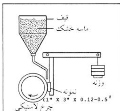
شکل ۲- نمایی از آزمون سایش خراشان بر اساس معیار ASTM G65.
