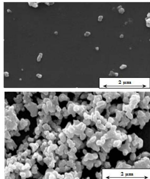
شکل ۵- مورفولوژی پودر YSZ8 در بزرگنمایی‌های مختلف
