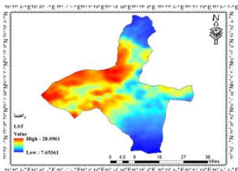
شکل (۲): نقشه دمای سطح زمین (LST) شهرستان تبریز برای سال‌های ۲۰۱۴-۲۰۲۳
