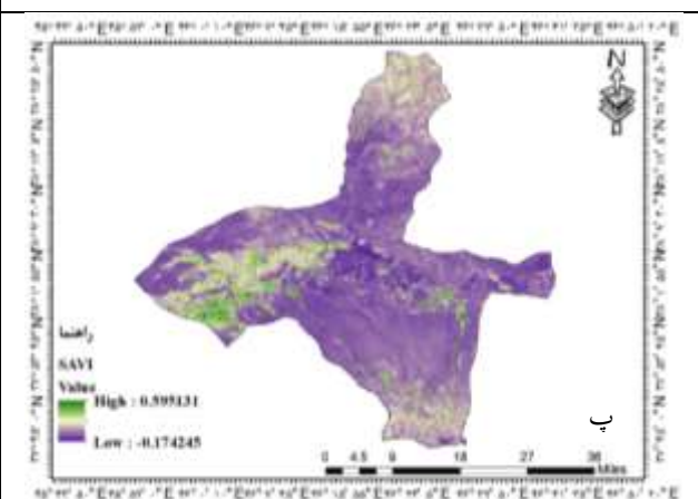
شکل (۷): نقشه میانگین شاخص SAVI شهرستان تبریز طی سال‌های ۱۳۹۳-
