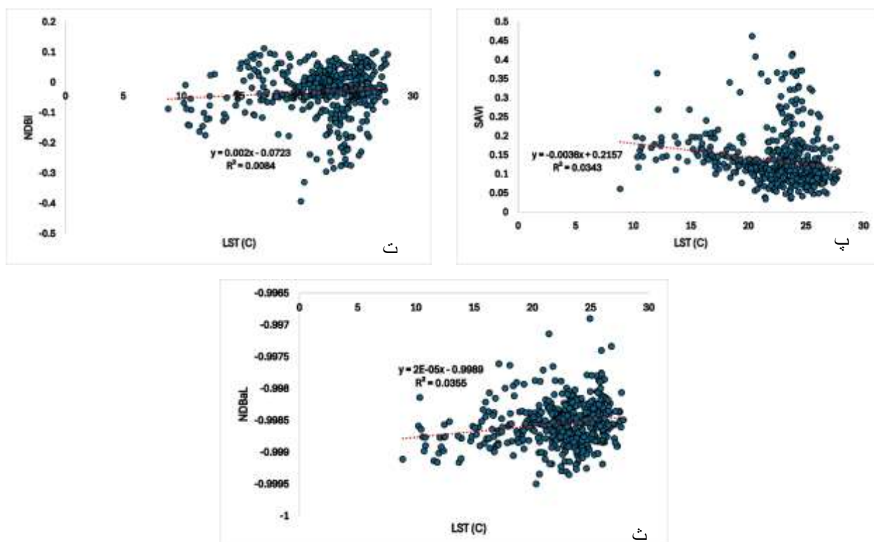
شکل (۹): نمودار ضریب تبیین شاخص LST با شاخص‌های طیفی (الف) NDVI، (ب) SAVI، (ت) NDBI، (ث) NDBaL شهرستان تبریز برای سال‌های ۲۰۱۴-۲۰۲۳
