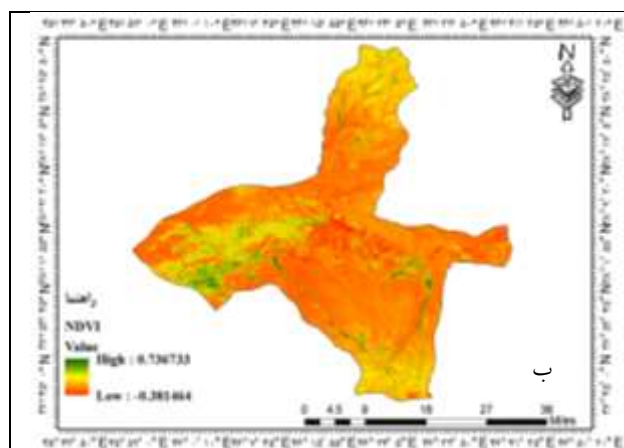
شکل (۴): نقشه میانگین شاخص NDVI شهرستان تبریز طی سال‌های ۱۳۹۳-
