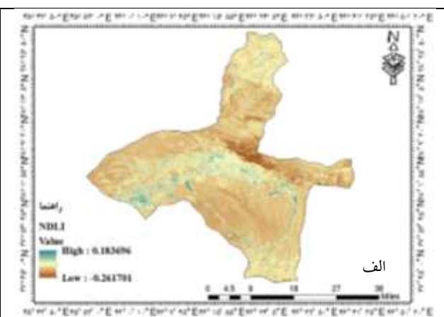
شکل (۵): نقشه میانگین شاخص NDLI شهرستان تبریز طی سال‌های ۱۳۹۳-
