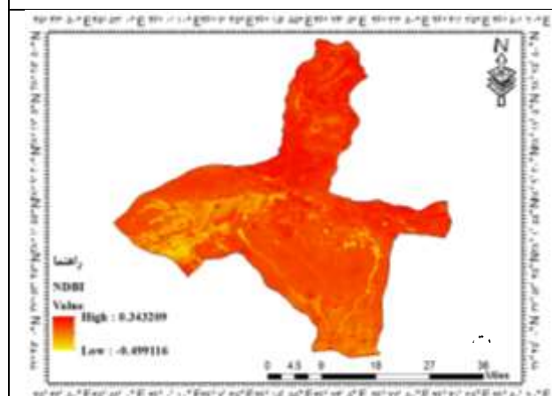
شکل (۶): نقشه میانگین شاخص NDBI شهرستان تبریز طی سال‌های ۱۳۹۳-
