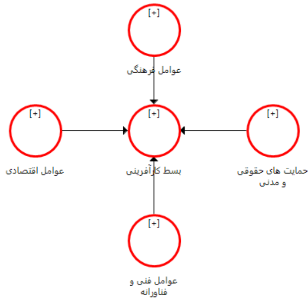
شکل (۴)، مدل برازش شده
