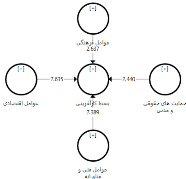
شکل (۱)، ضرایب معناداری در مدل
