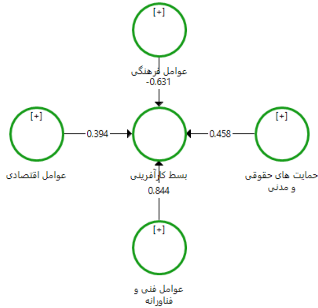
شکل (۳)، خروجی ضرایب استاندارد مسیر
