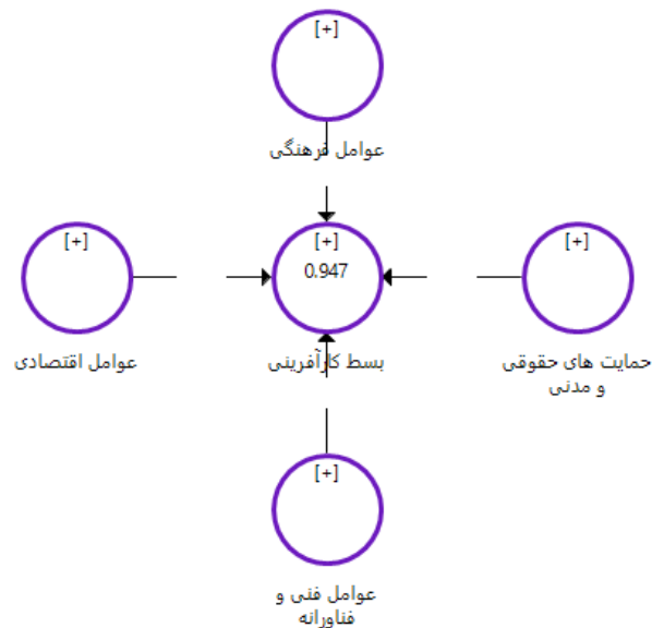
شکل (۲)، ضرایب R^2 ویژه متغیرهای درون‌زای مدل
