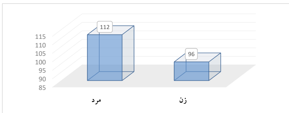
نمودار ۱- فراوانی متغیر جنسیت
