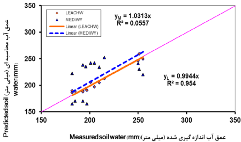
شکل ۸- مقایسه نتایج تخمین زده شده و مشاهده‌ای عمق آب پروفیل خاک با خط یک به یک با استفاده از دو مدل MEDIWY و
