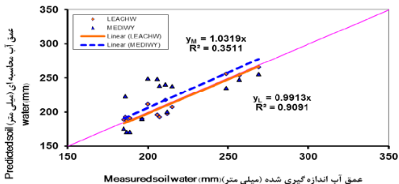
شکل ۹- مقایسه نتایج تخمین زده شده و مشاهده‌ای عمق آب پروفیل خاک با خط یک به یک با استفاده از دو مدل MEDIWY و
