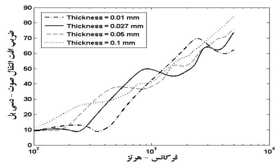
شکل (۸) اثر ضخامت لایه متخلخل بر TL در حالت (B-U).
