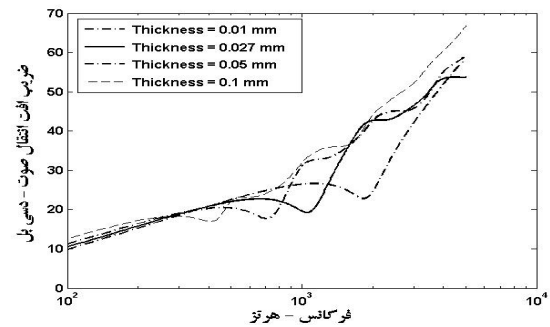
شکل (۹) اثر ضخامت لایه متخلخل بر TL در حالت (B-B).
