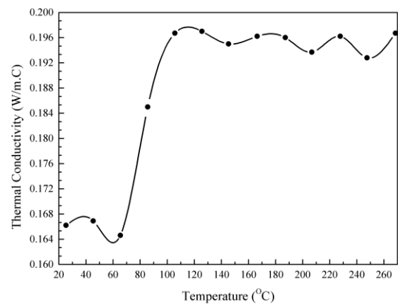
شکل (۳) ضریب انتقال حرارت PMMA.
