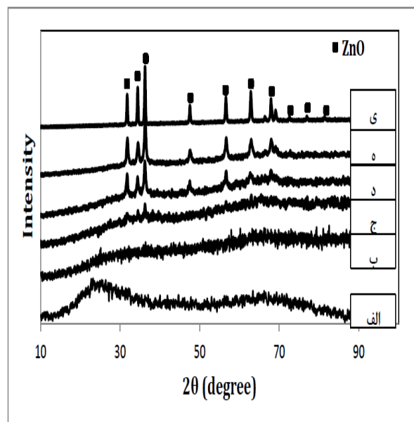
شکل (۲): الگوی پراش اشعه ایکس در دمای ثابت از نمونه های: (الف): ۱۰۰Z (ب): ۳۰ZAS، (ج): ۴۰ZAS، (د): ۵۰ZAS، (ه): ۷۰ZAS و
